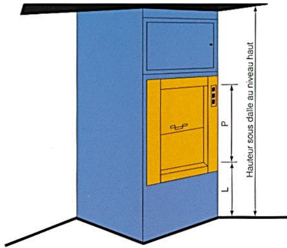
Portes à guillotine sur allège
