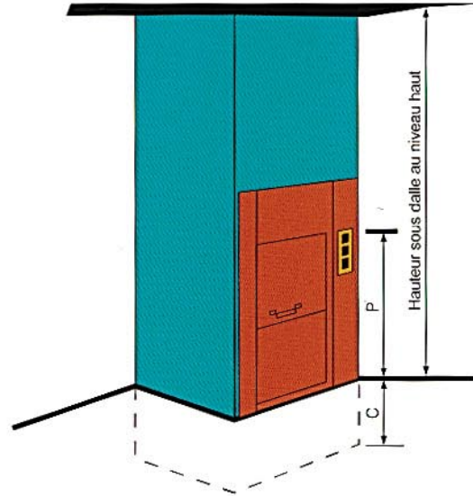
Portes à guillotine au ras du sol
